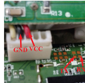
Fig. 8. UART of WeMo plug.
